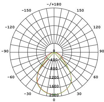
CURVA FOTOMETRICA
